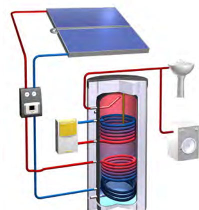
Production de chaleur : schéma d'un chauffe-eau solaire
